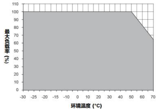
图 1 ) 温度降额_ 输出负载降额对应环境温度
