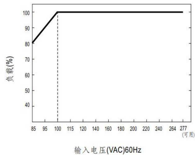
图 2 ) AC 输入电压降额_ 输出负载降额对应输入电压
