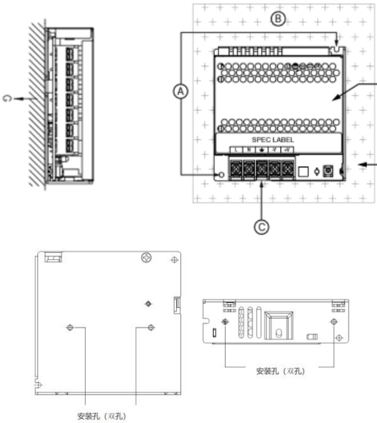
图. 3.2 安装位置
